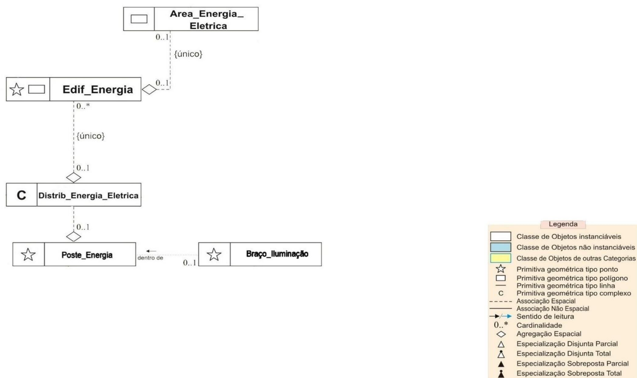
Figura 6. Diagrama de classe da categoria Energia das áreas urbanas do município de Cáceres. Adaptado de BRASIL, 2007.
