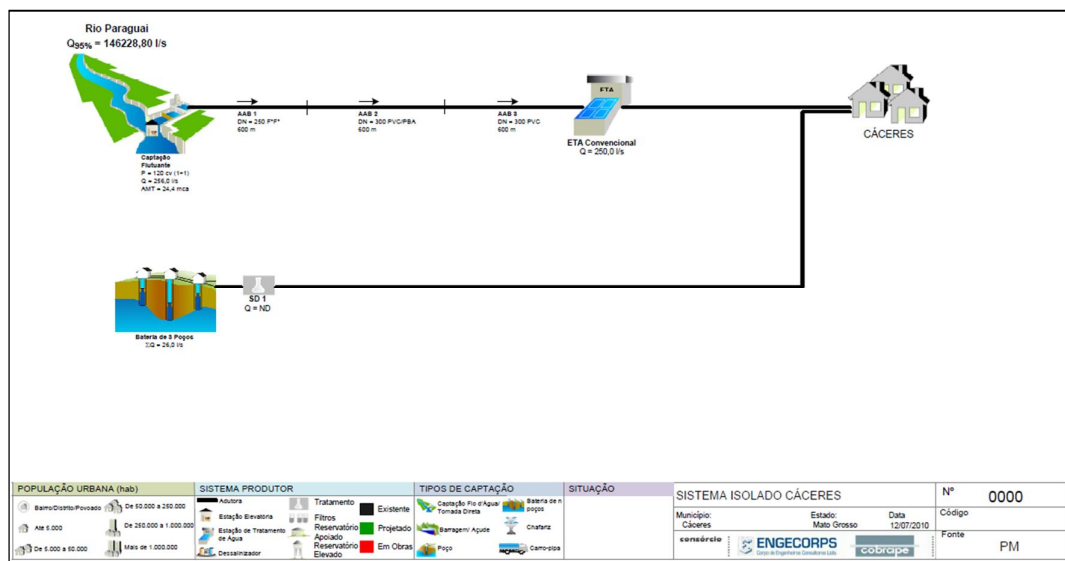
Figura 19. Esquema do sistema de abastecimento de água de Cáceres-MT. Fonte: Ana (2010).
