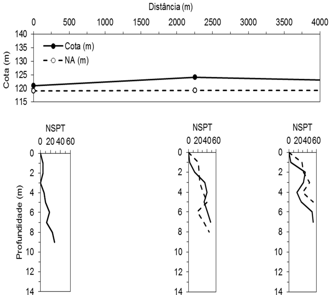
Figura 14. Perfil de solo em Cáceres-MT - Perfil 02: SPT-02, SPT-07 e SPT-08
